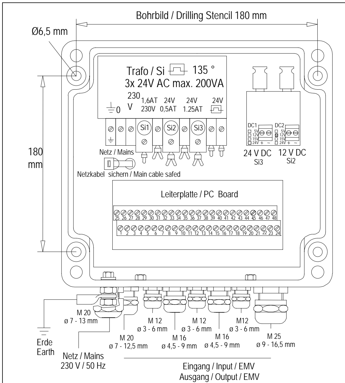
„Layout / Bohrbild“ / ..Layout/Drilling template.
